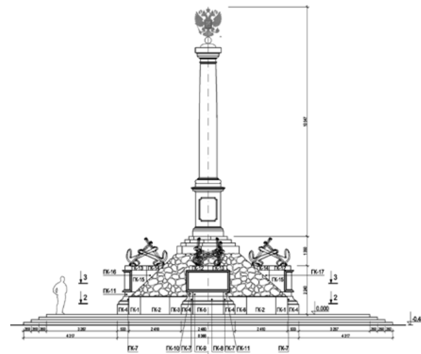
Чертеж фасада из проекта стелы для города воинской славы Кронштадт, общий вид готового сооружения и барельефы его скульптурного декора
